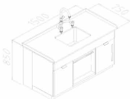
IM9 шкаф с мойкой 1500л
