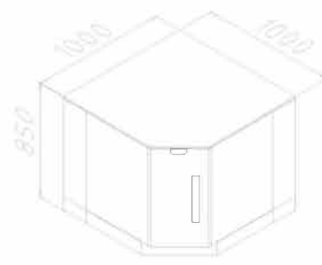
Чертеж углового шкафа IM9
