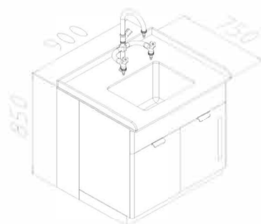
Шкаф IM9 с мойкой 900л
